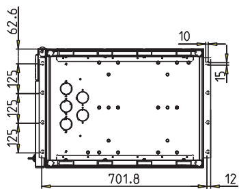
底视图
