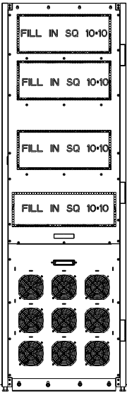
后视图
