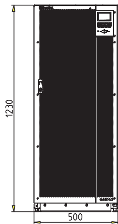
前视图
