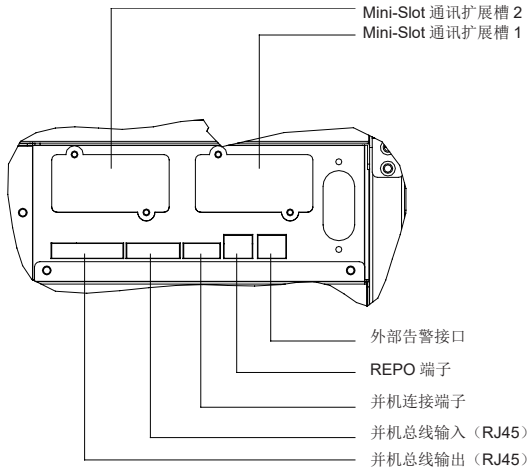
15KS-40KS 通讯接口位置图:
