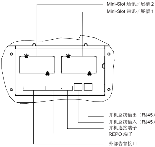
60KS-100KS 通讯接口位置图:
