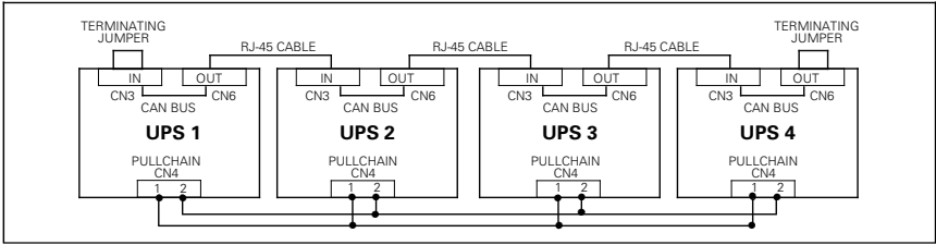
并机接线图-不带并机柜
