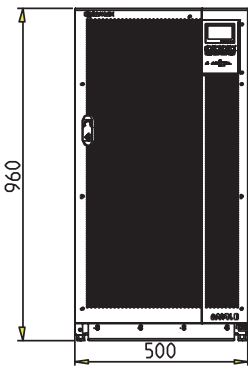
前视图
