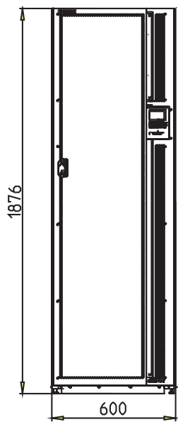
前视图
