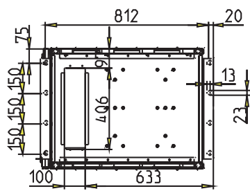
底视图
