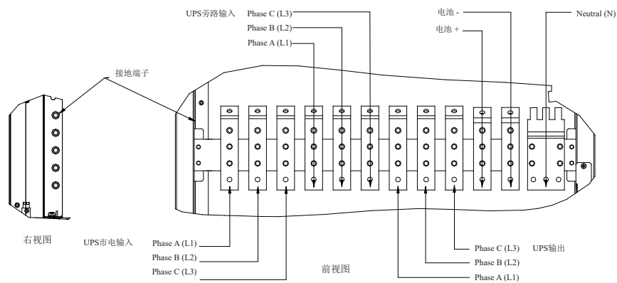
用户功率端子位置安装图:
