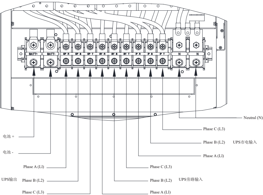
用户功率端子端子位置安装图:
