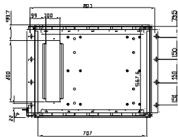
底视图
