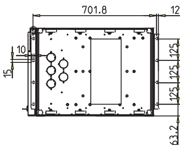
底视图
