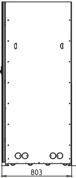
右视图
