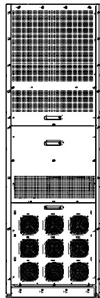
后视图
