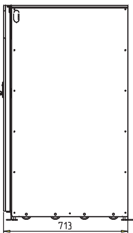
右视图
